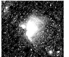
オリオン座大星雲
